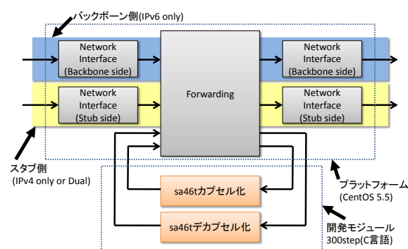
図 3: SA46T の実装構成
